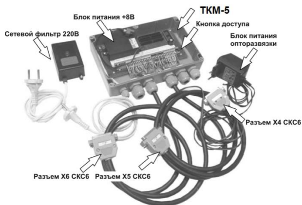
Рис. Д.2 Схема поверки ВКГ-2 с использованием СКС-6 и ТКМ-5 Разъемы X4...X6 (ТКМ-5) подключаются к одноименным разъемам стенда СКС6
